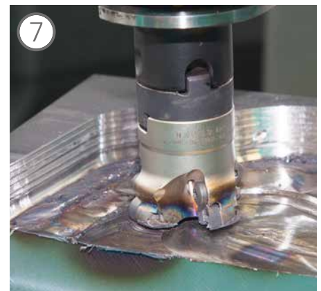
Risultato: gravi danni a utensile e pezzo
