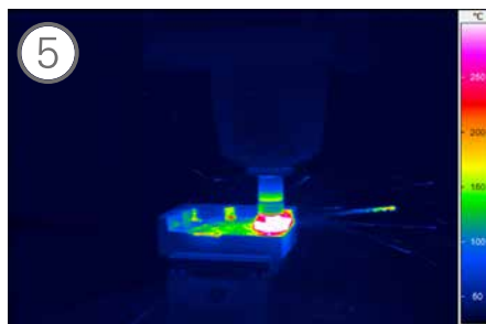
Oltre il campo di misura: la temperatura della fresa a inserti supera i 300 °C.
