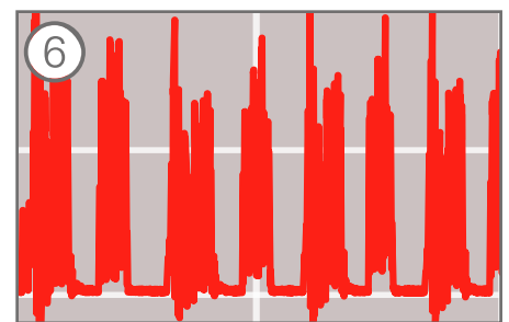
Poco prima dell'arresto d'emergenza: potenza assorbita dal mandrino con funzione AFC disattivata
