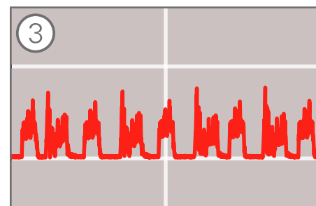
3 Dopo 58 minuti con AFC: potenza assorbita dal mandrino all'arresto della lavorazione da parte di AFC
